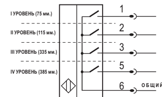
Схема подключения
